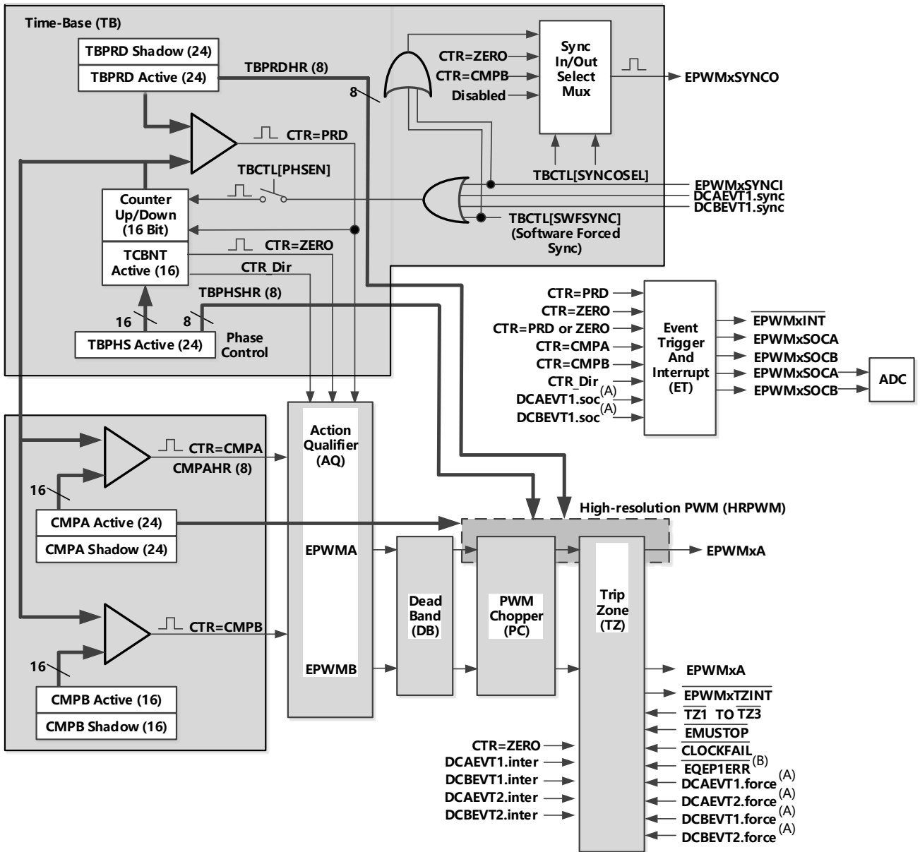
图 4-13 ePWM 子模块显示关键内部信号互连
