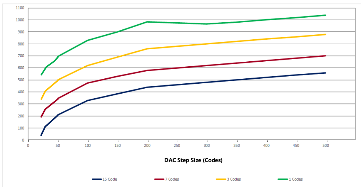
图 6-24 DAC 设置时间
