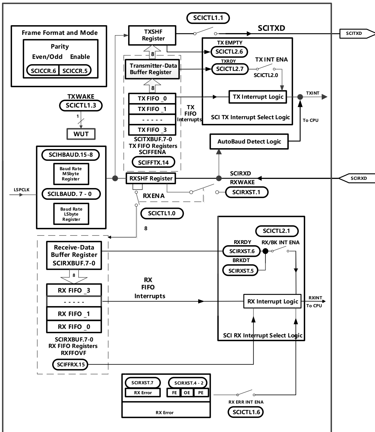
图4-7 串行通信接口(SCI) 模块方框图
