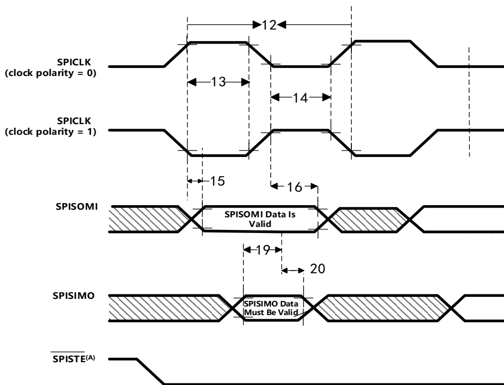
图6-22 SPI 受控模式外部时序 (时钟相位= 0)
