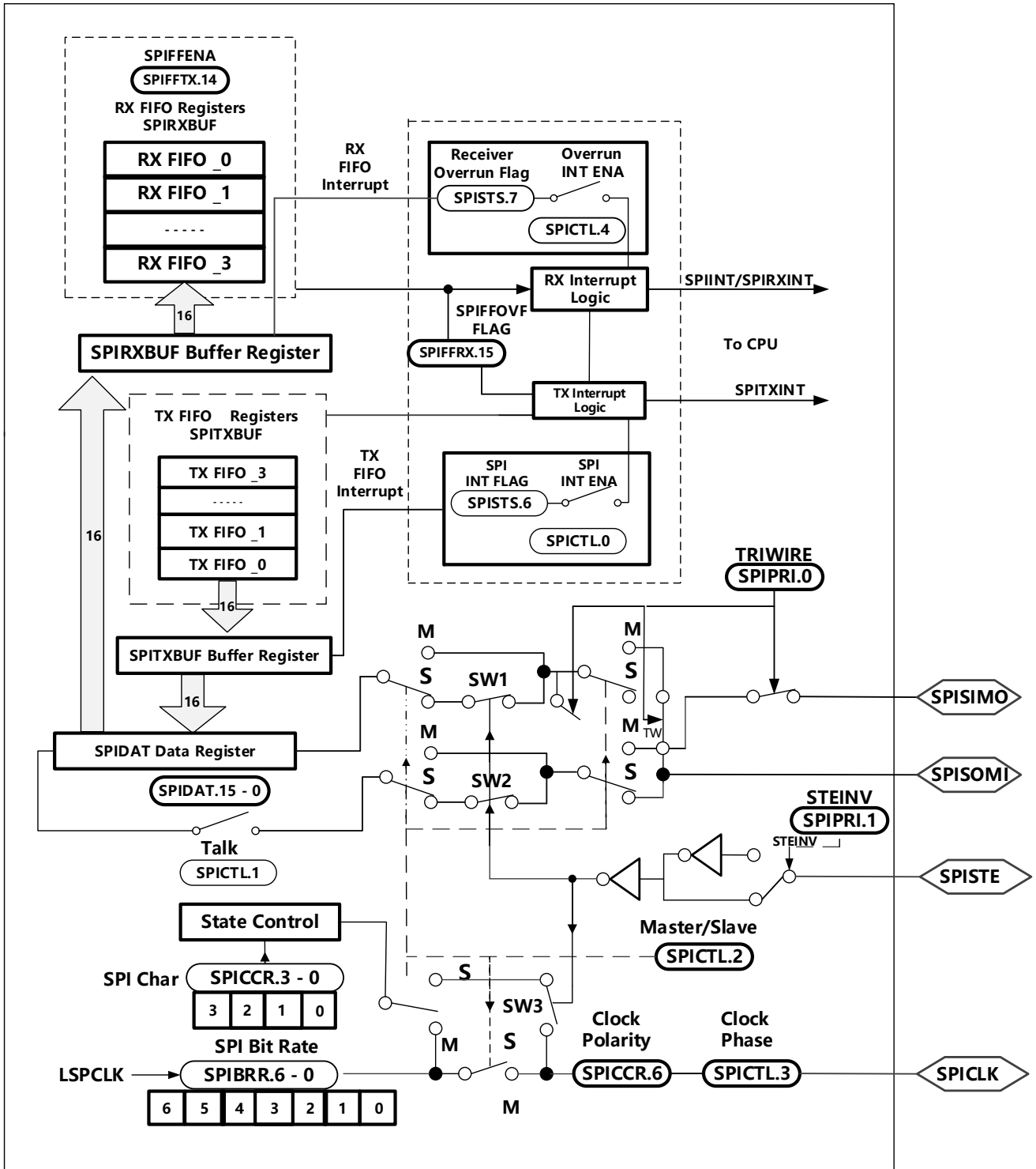
图4-6是一个处于受控模式下的SPI的方框图。
