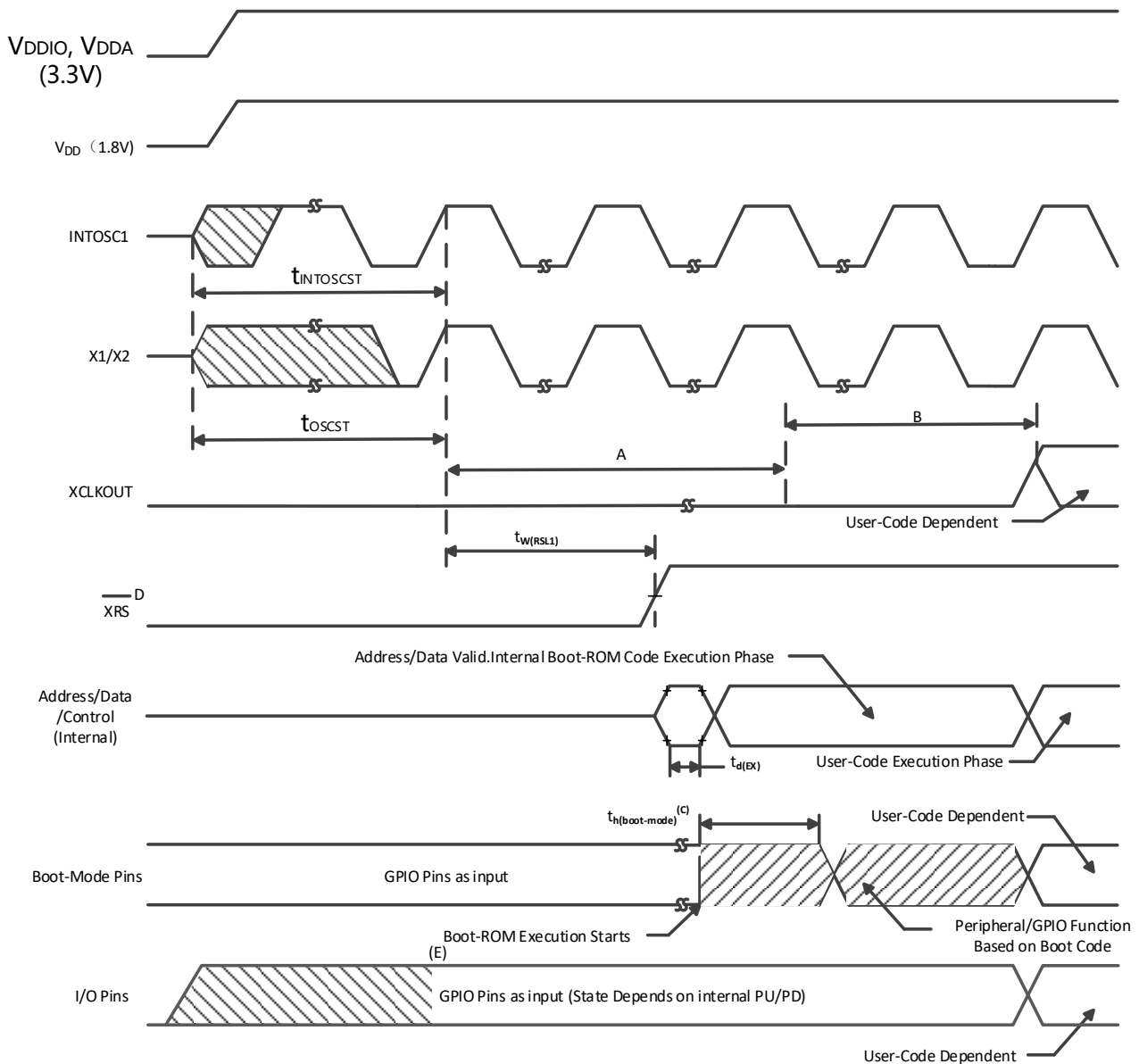
图6-7 加电复位
