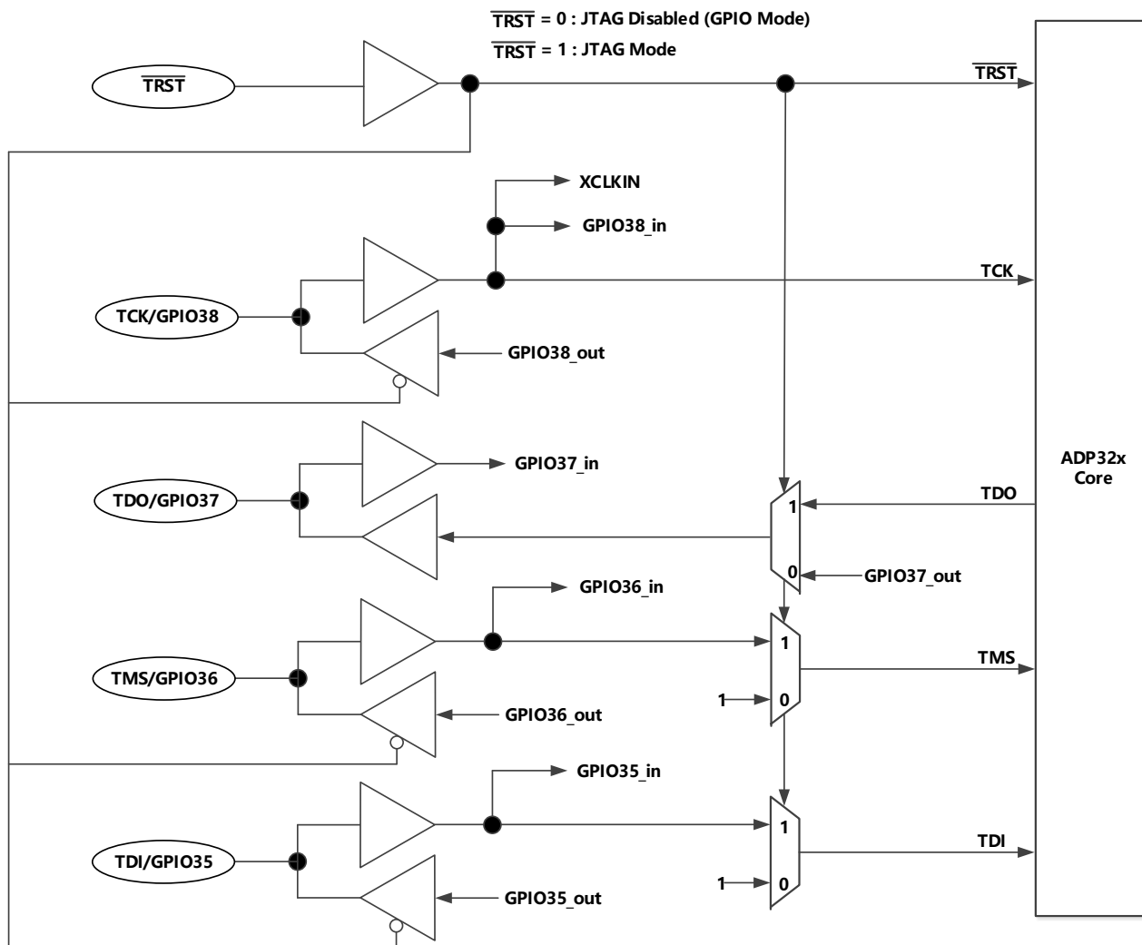
图 4-17 JTAG/GPIO 复用
