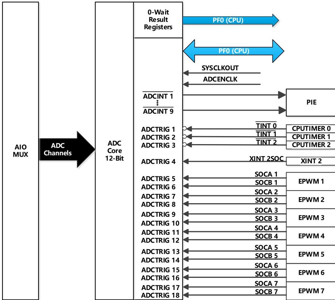
图 4-3 ADC 连接
