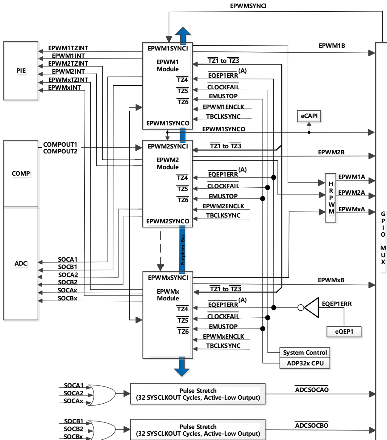
图 4-12 ePWM
