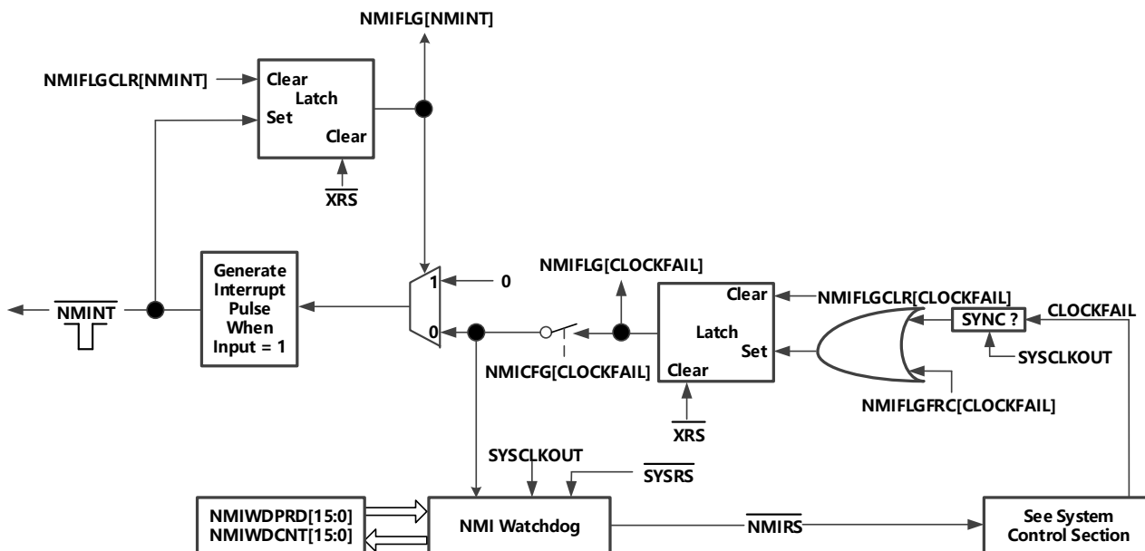
图 3-10 NMI - 看门狗
