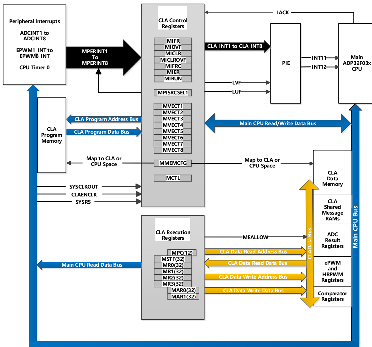
图 4-1 CLA 方框图
