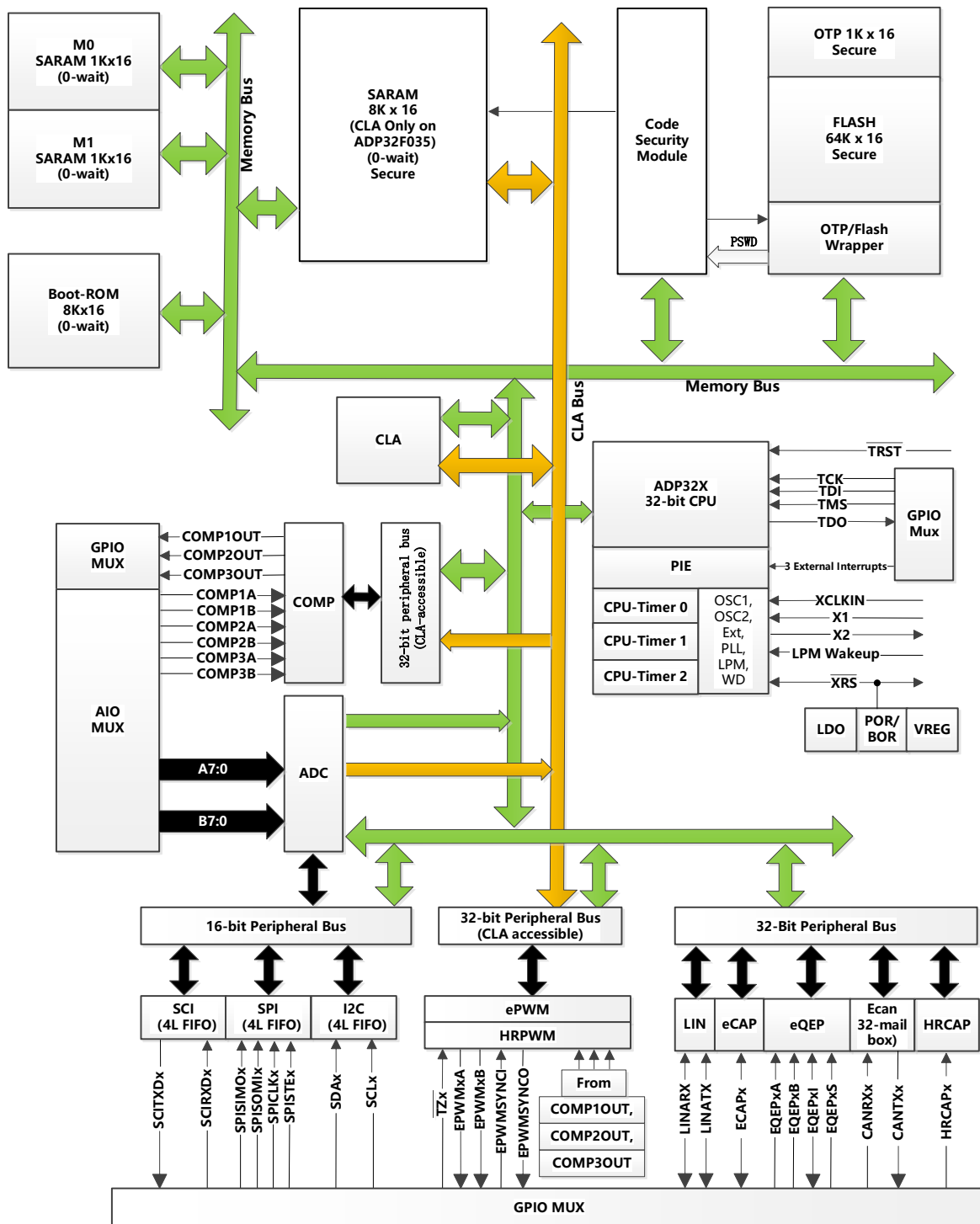
图 3-1 功能方框图
