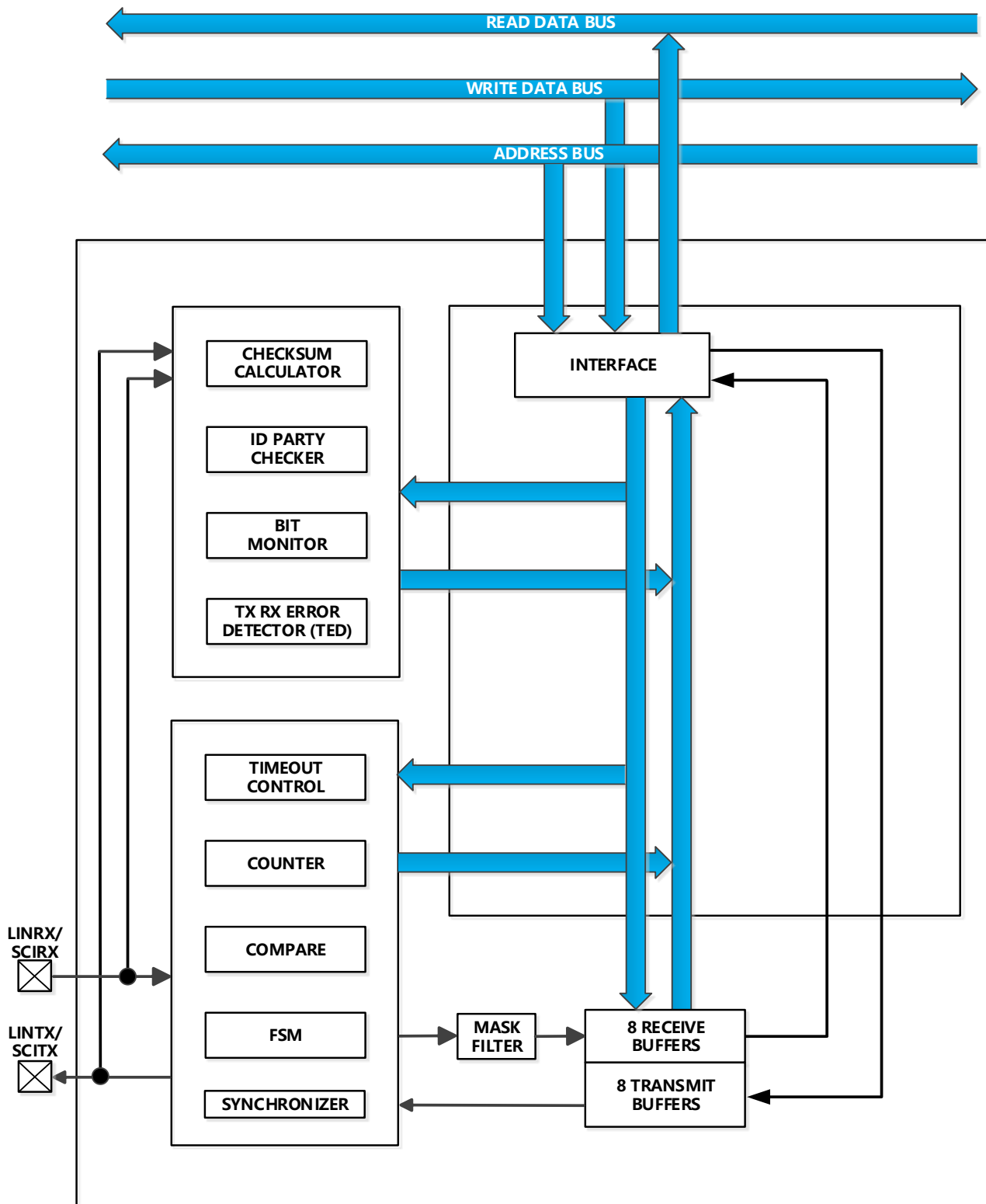
图 4-8 LIN 方框图
