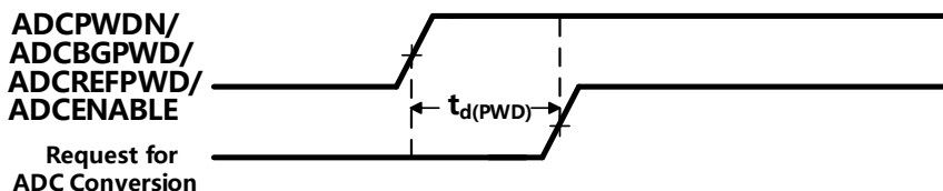
图6-25 ADC 转换时序
